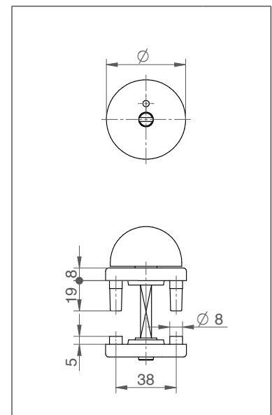
WC-Drehknopf
