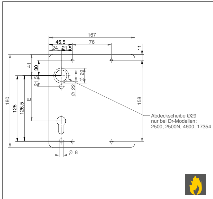
Breitschild, Schildstärke 8 mm, Bohrloch: \varnothing 8,2 mm D55
