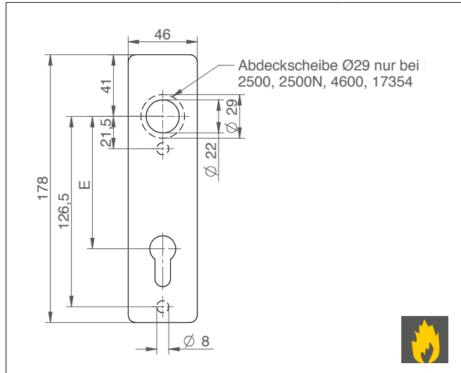
Kurzschild eckig, Schildstärke 8 mm, Bohrloch \varnothing 8,2 mm D52
