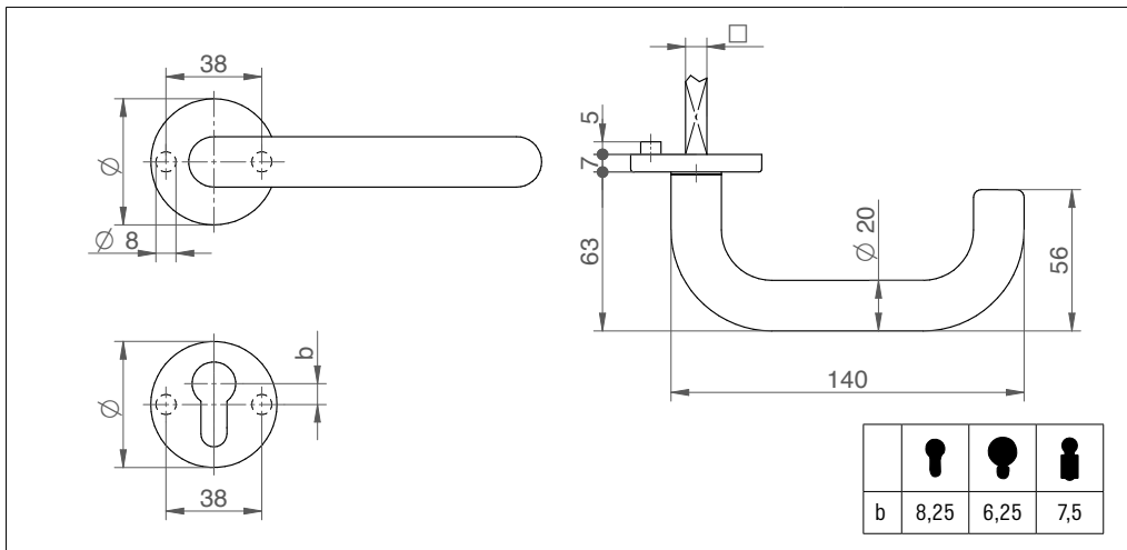
Rosettendurchmesser 50 mm \varnothing , Rosettenhöhe 7 mm
