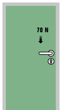
Innenseite EN 179
