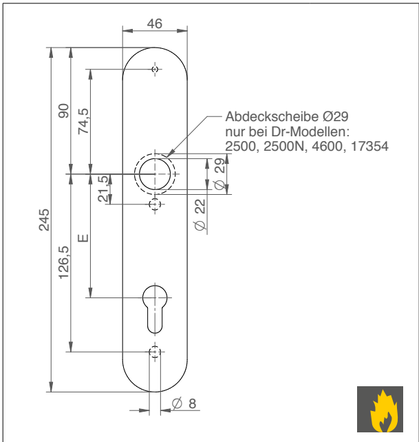
Langschild abgerundet, Schildstärke 8 mm, Bohrloch: \varnothing 8,2 mm D53
