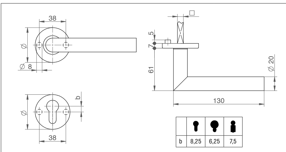
Rosettendurchmesser 50 mm \varnothing , Rosettenhöhe 7 mm
