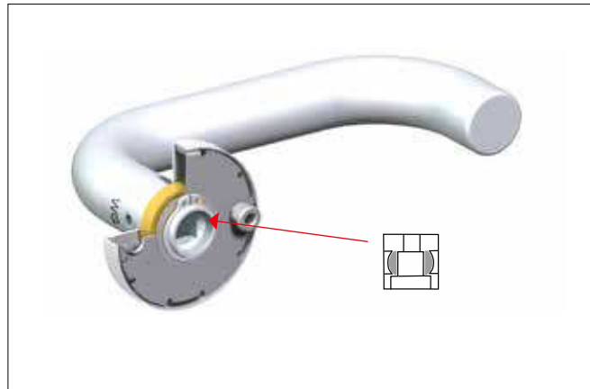
WG4-Rosette mit Metallgleitlager
