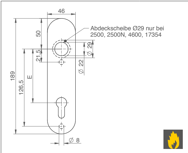
Kurzschild abgerundet, Schildstärke 8 mm, Bohrloch \varnothing 8,2 mm D51
